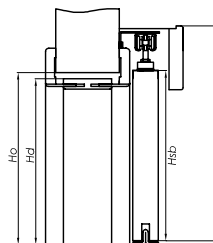
drzwi przesuwne – system naścienny z zabudową tunelową ZN
