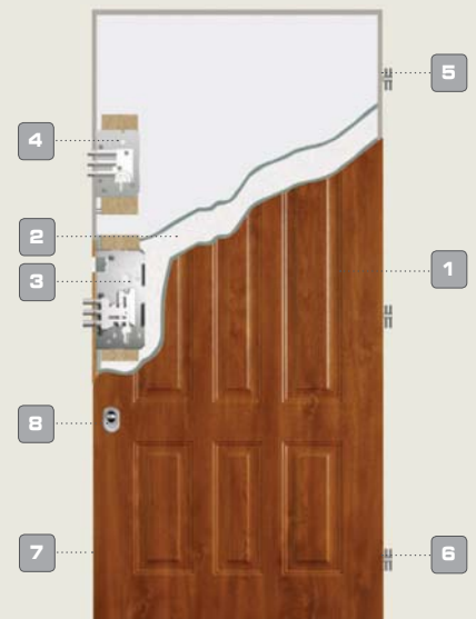
GRUBOŚĆ SKRZYDŁA 57 mm
