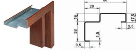
OŚCIEŻNICA NAROŻNIKOWA BEZ USZCZELKI FN (do drzwi TT i GTT)
